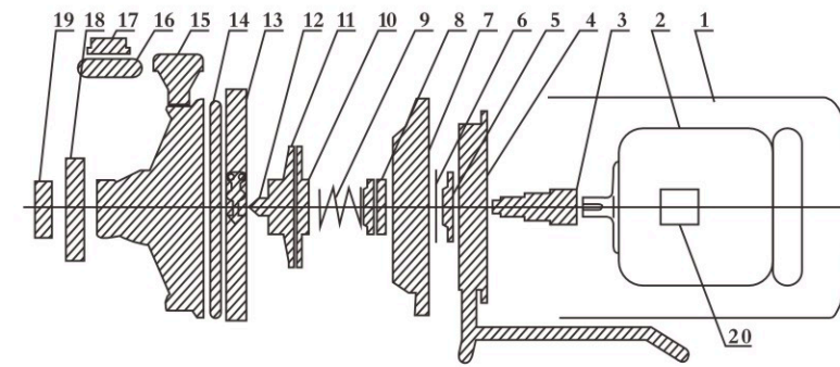
BAW-150型不锈钢卫生泵结构图
